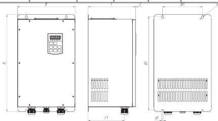
Рис. 2.7 Габаритные и установочные размеры устройств серии LCI в корпусе IP54
