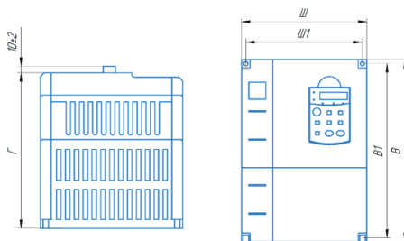
Рис. 2.5 Габаритные и установочные размеры устройств серии LCI в пластмассовом корпусе
