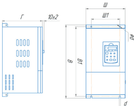
Рис. 2.6 Габаритные и установочные размеры устройств серии LCI в металлическом корпусе
