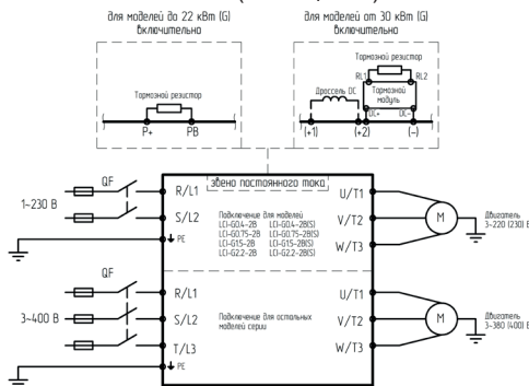
Рис. 3.2. Схема силовых подключений для серии LCI и LCI (S)
